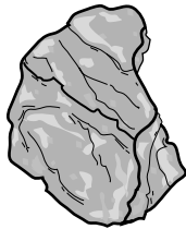
Magnetite
