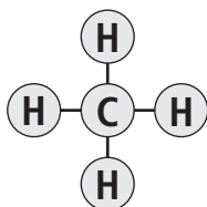
\text{CH}_4
